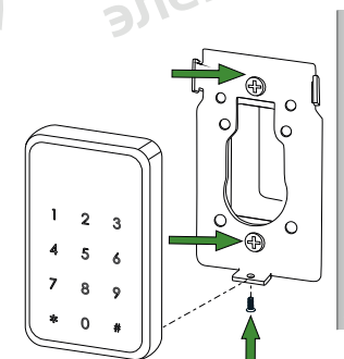
Рисунок №2.2 – Установка считывателя-контроллера
