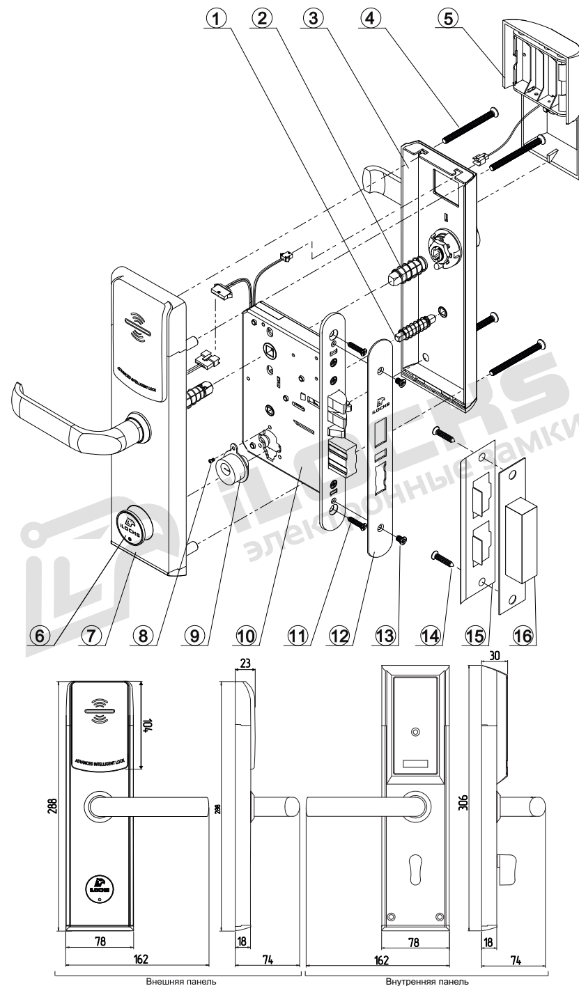
Рисунок №1 – Структурная схема (спецификация) и габариты замков типа iLOCKS IS8005AB3 433+BLE
