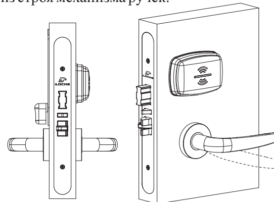
Рисунок №8 - Крепление внешней и внутренней ручек
