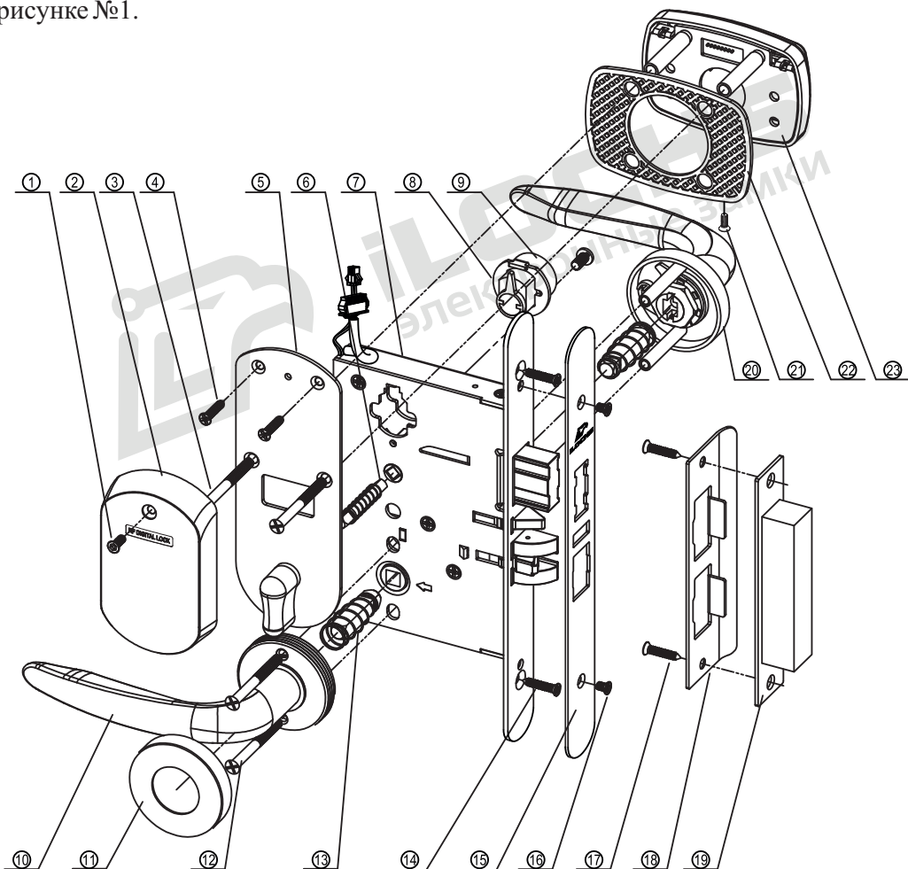
Рисунок №1 – Структурная схема (спецификация) замков типа iLOCKS IS100 433+BLE
