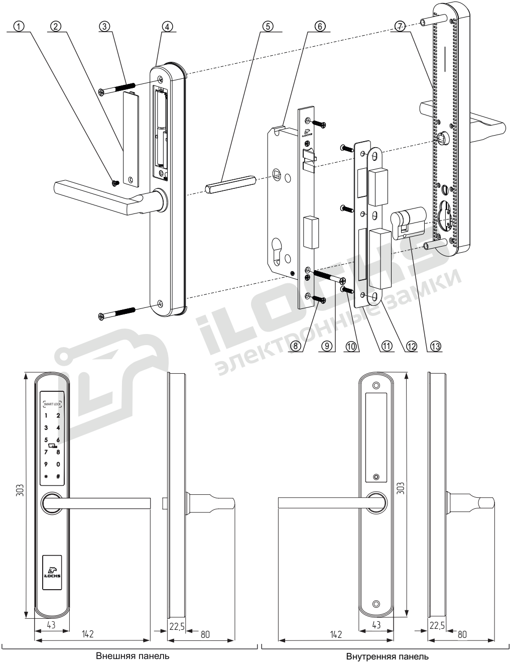
Рисунок №1 – Структурная схема (спецификация) и габариты замков типа iLOCKS IS210AB-BL
