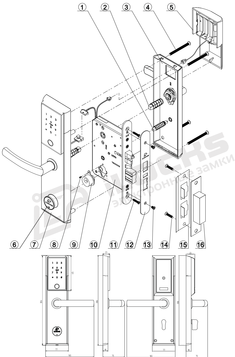
Рисунок №1 – Структурная схема (спецификация) замков типа IS8005AB3-BBL 433+BLE
