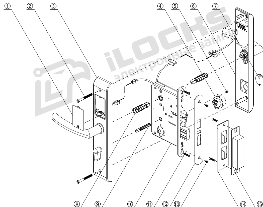
Рисунок №1 – Структурная схема (спецификация) замков типа iLOCKS IS201
