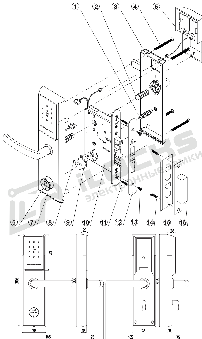
Рисунок №1 – Структурная схема (спецификация) и габариты замков типа iLOCKS IS8005AB3-BL
