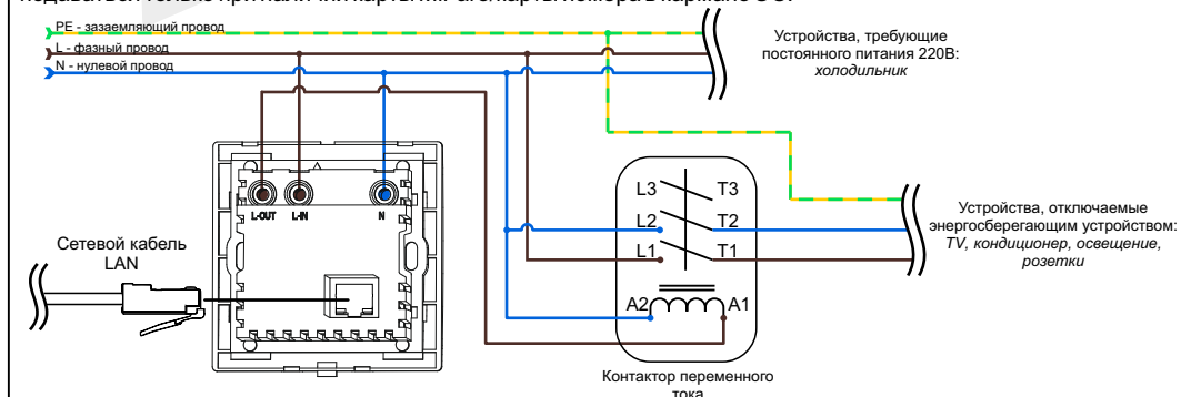
Рисунок 2. Схема подключения энергосберегающего устройства через контактор переменного тока
