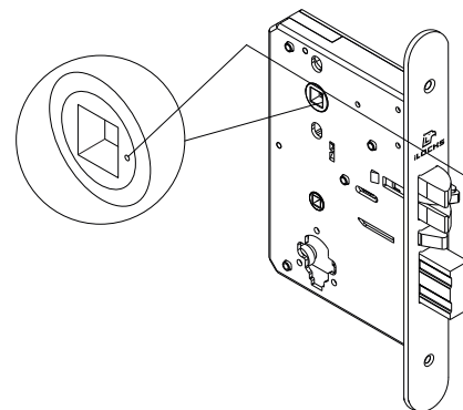
Рисунок №2.1 – Точка/стрелка. Точка на шпинделе должна находиться на уровне стрелки на корпусе врезного механизма замка.
