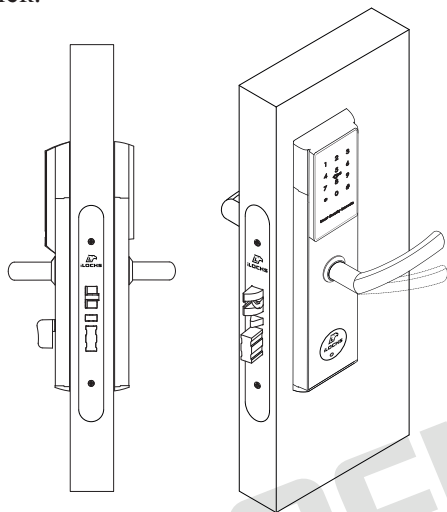
Рисунок №7 – Крепление панелей
