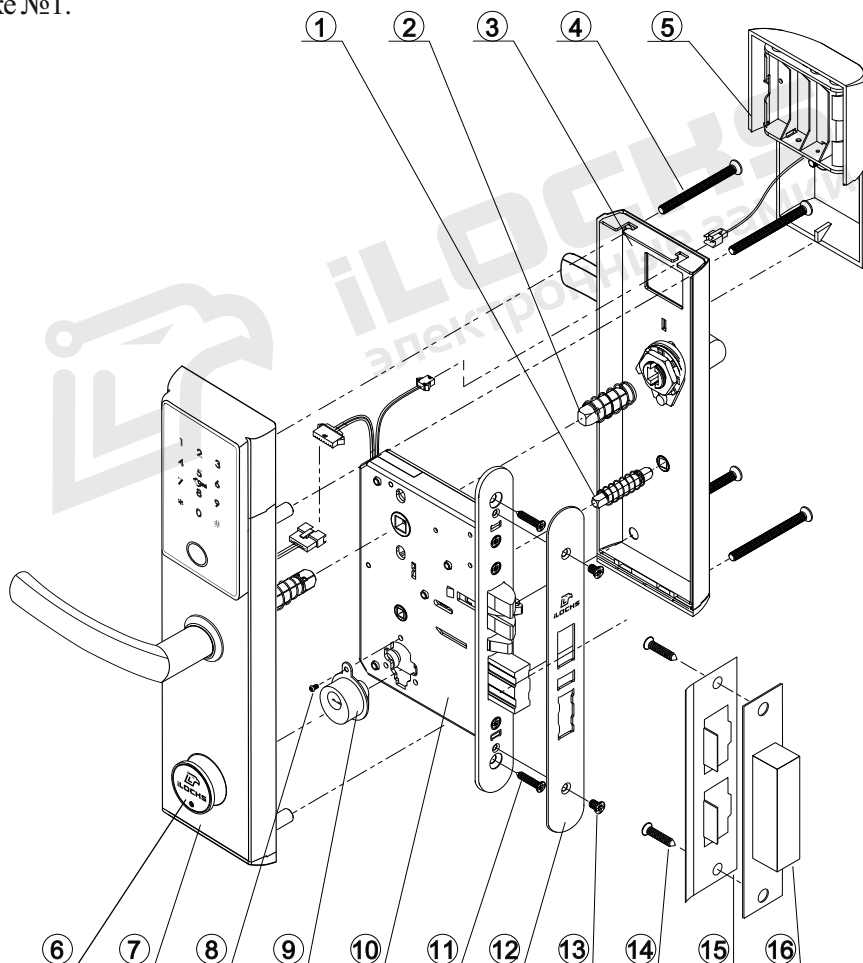
Рисунок №1 – Структурная схема (спецификация) замков типа IS8005AB3-BBL 433+BLE
